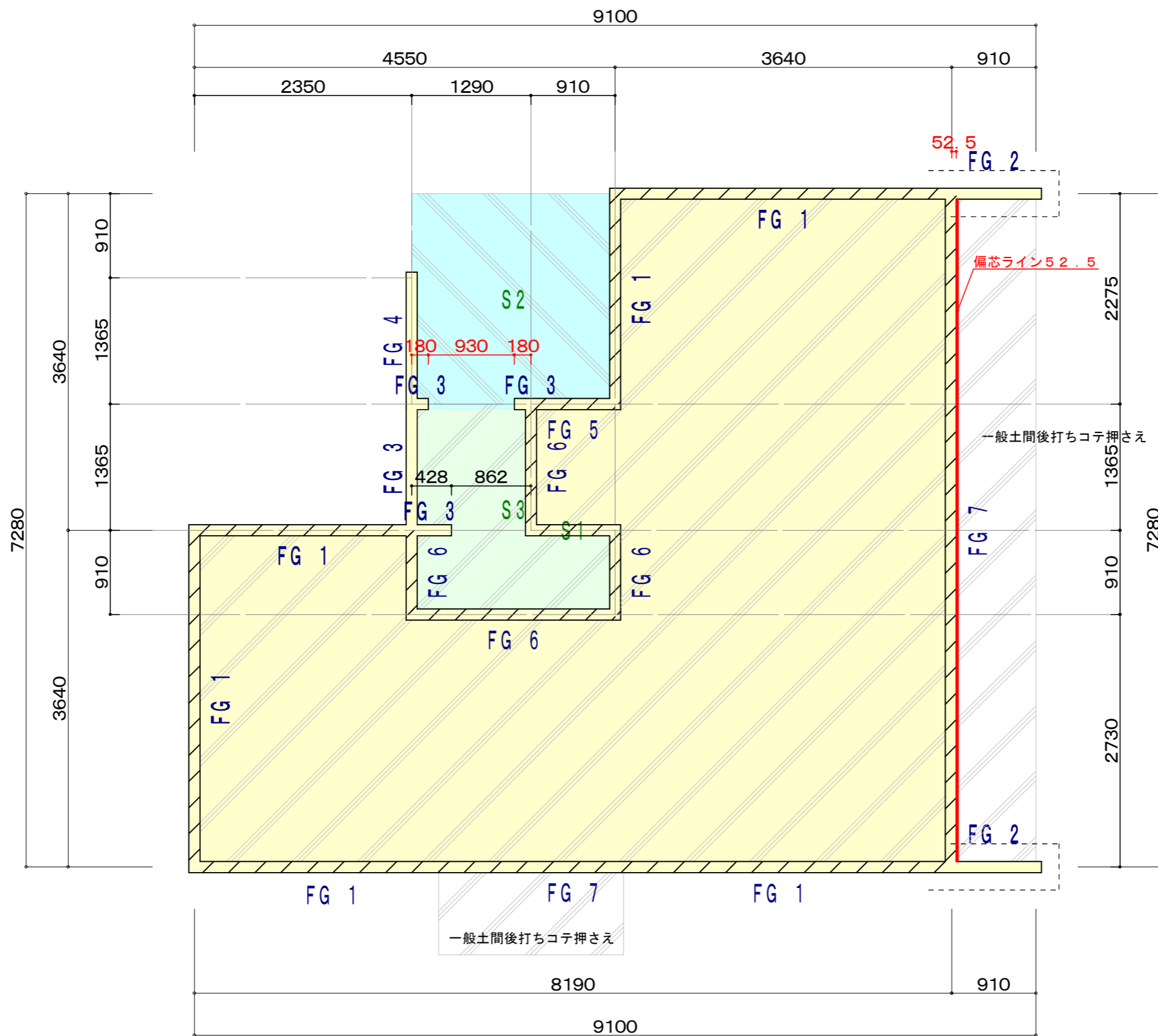
1階：基礎伏図
