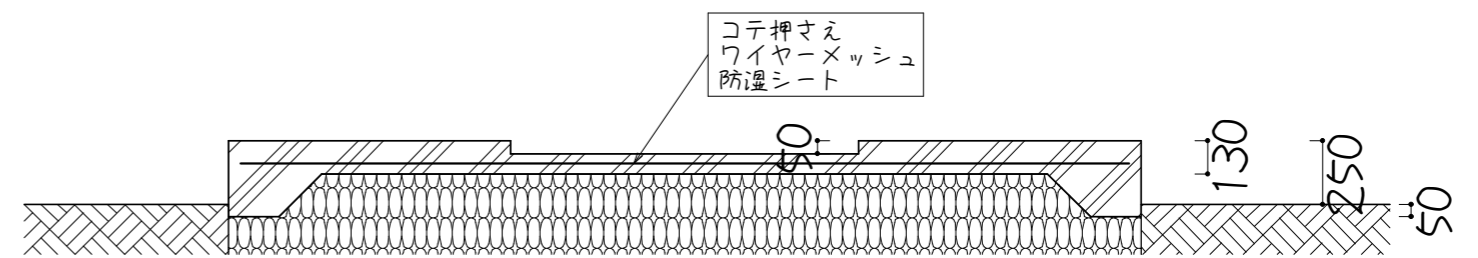
土間基礎 断面図
