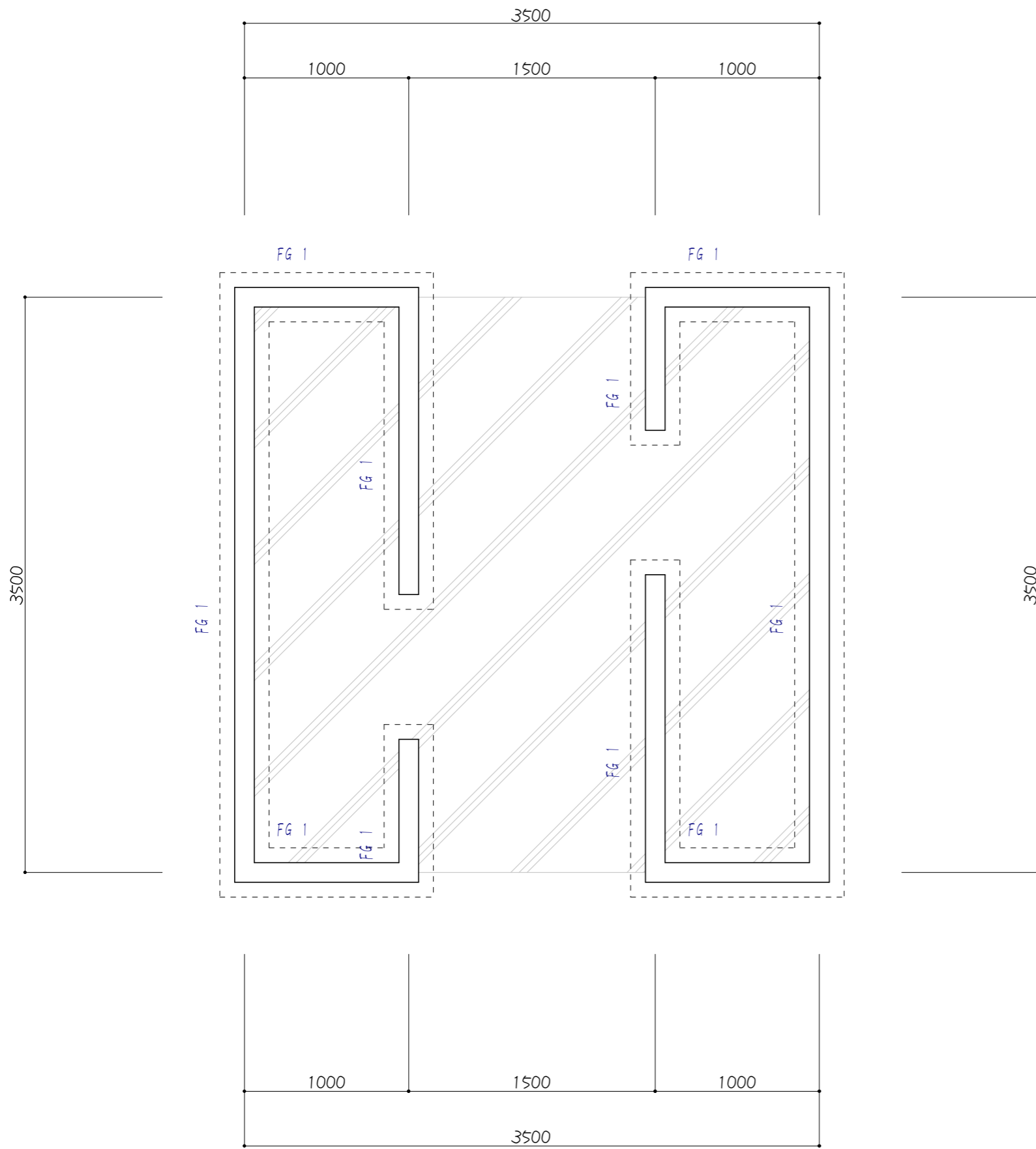
1階：基礎伏図
