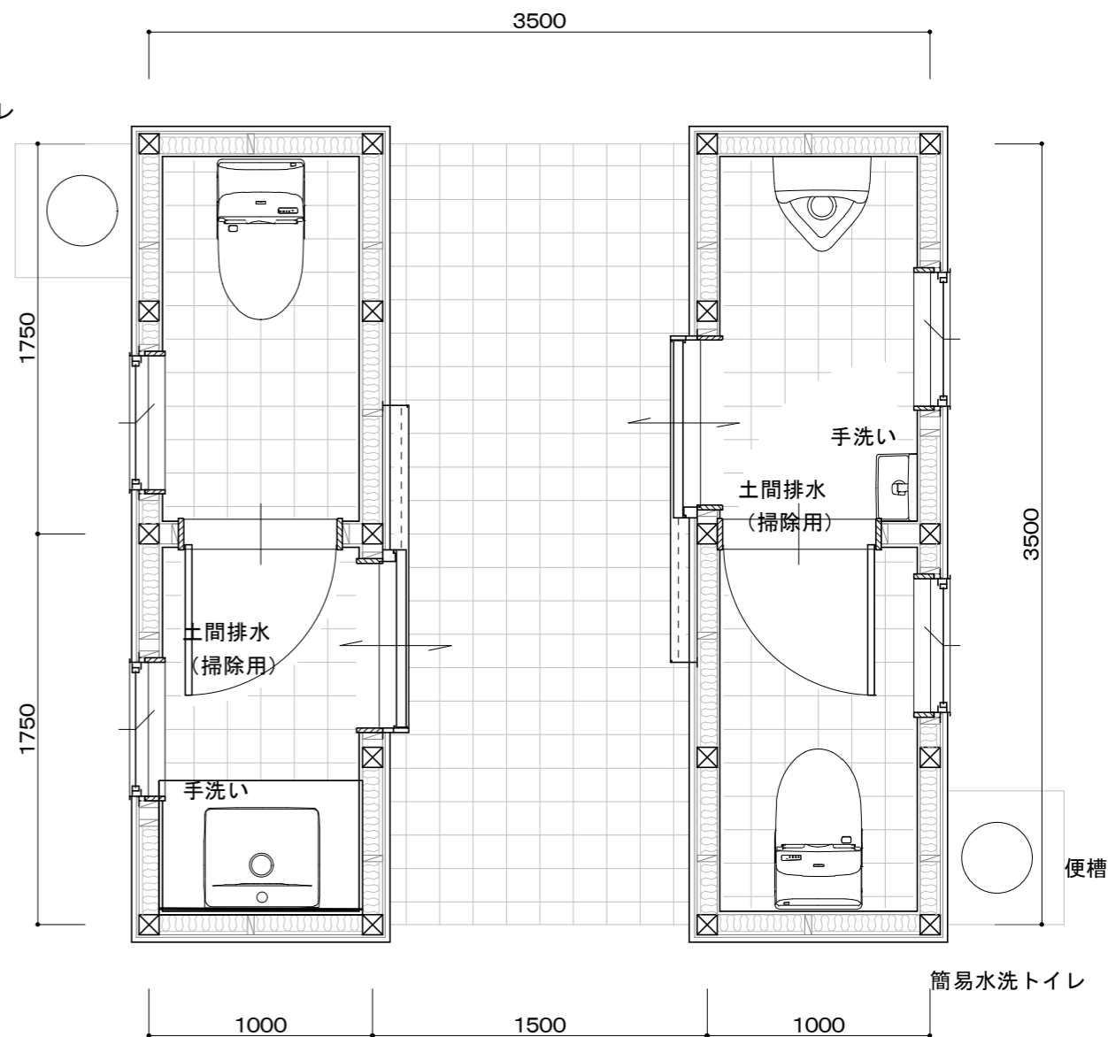
1/30 平面図
