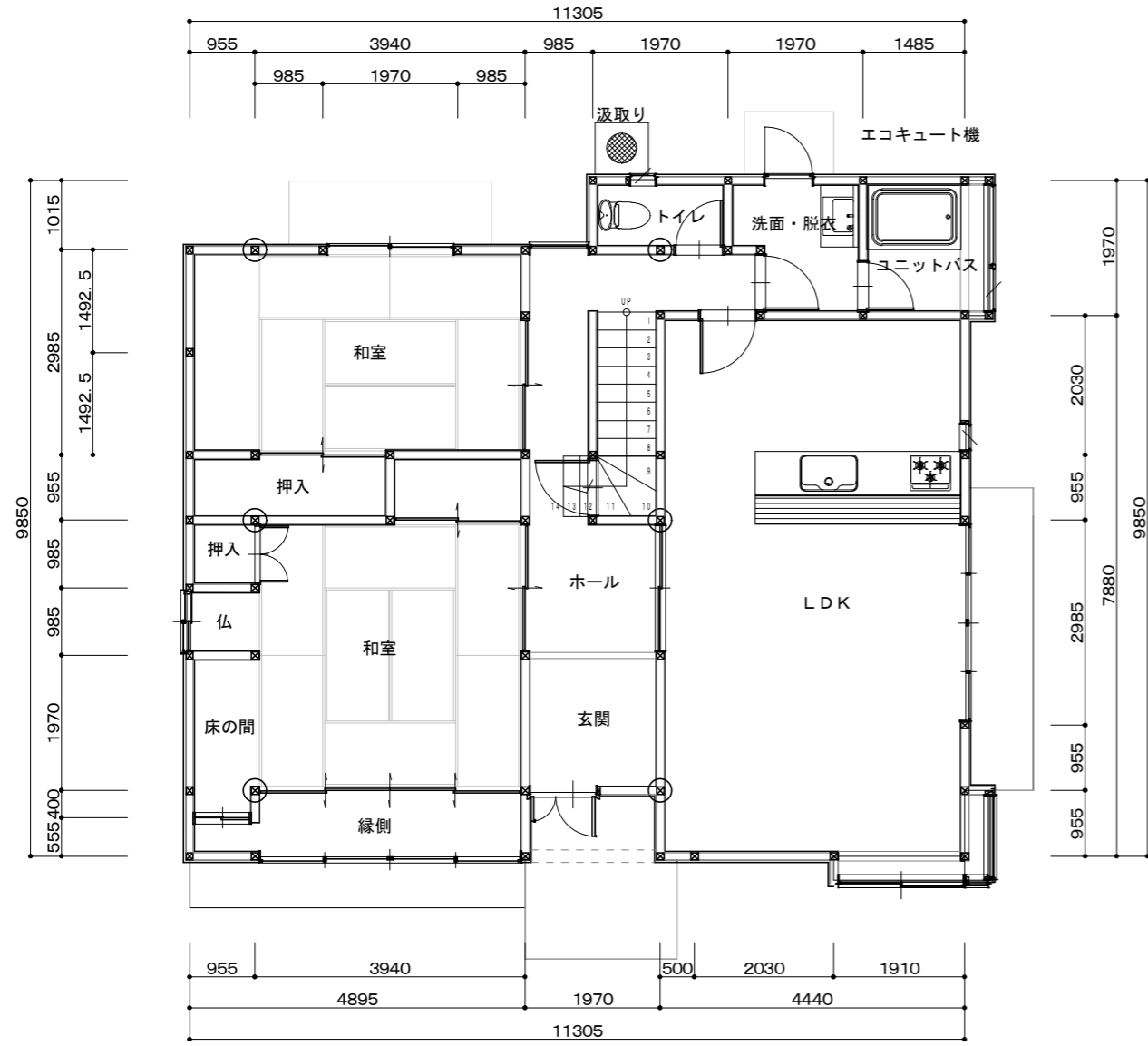
既存平面図 1 F
