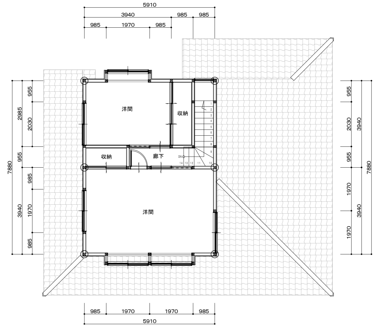
既存平面図 2 F
