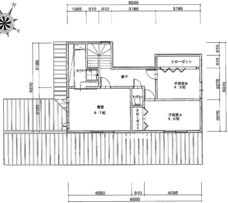
平面詳細図 2階
