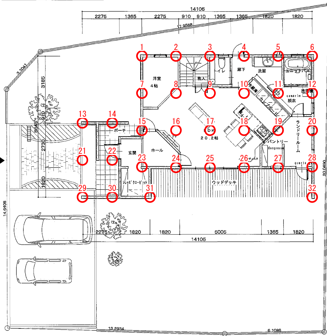
平面詳細図 1階
