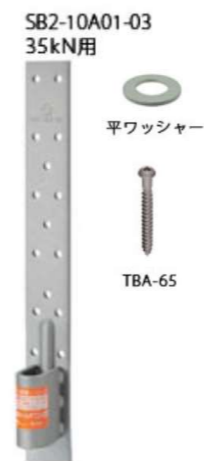
35kN用(使用本数15本)
