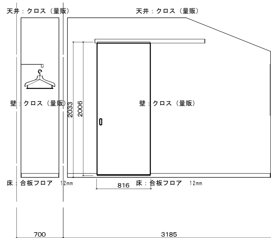
子供室B展開図
