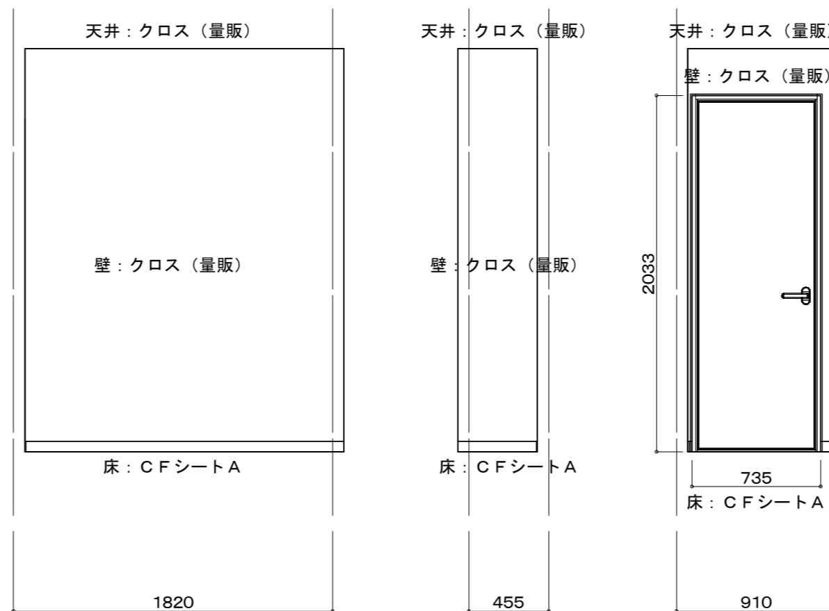
ランドリー展開図
