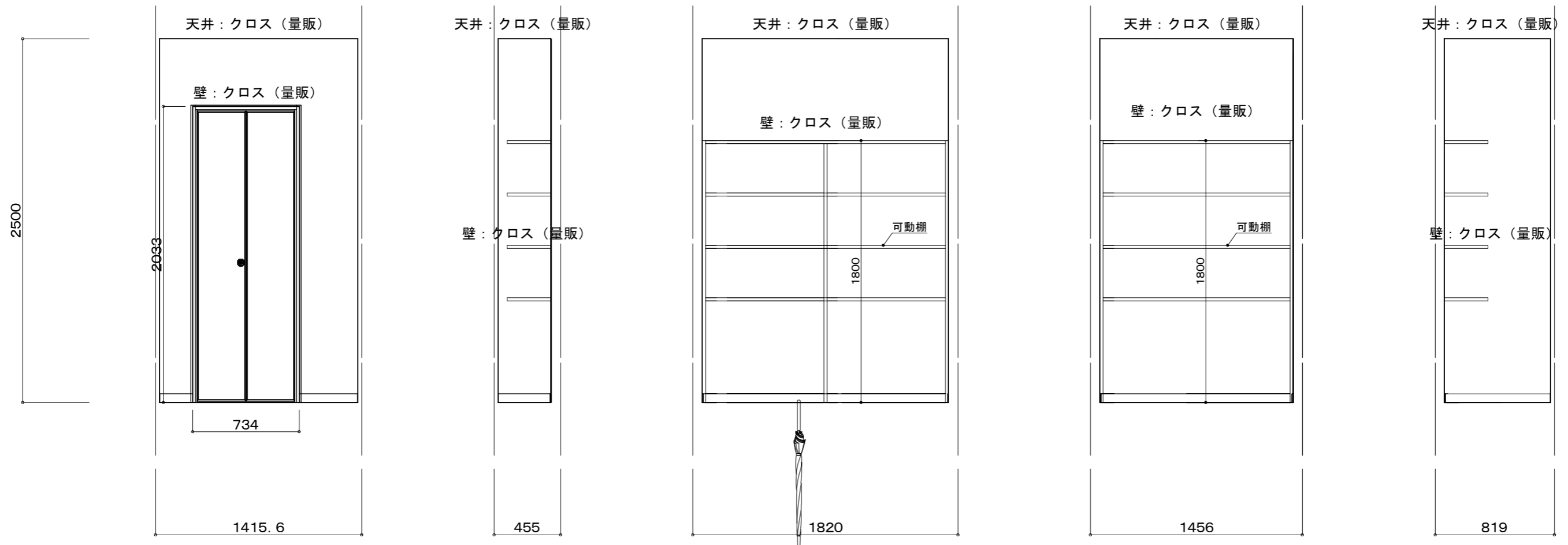
パントリー展開図
