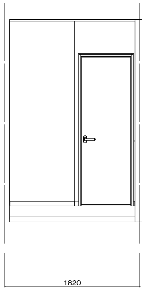
玄関展開図
