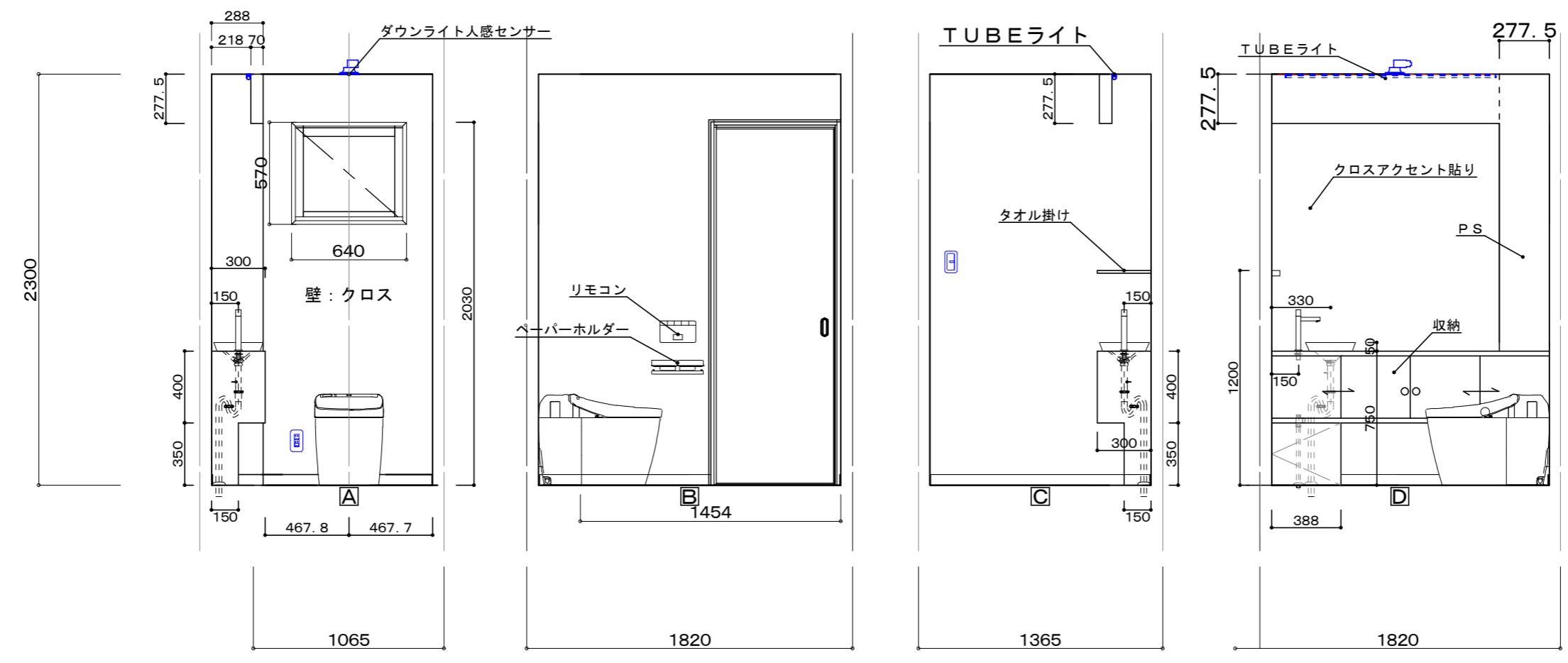
トイレ展開図
