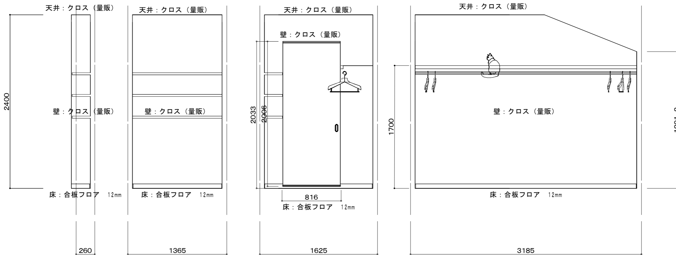
ウォークインクローゼット展開図
