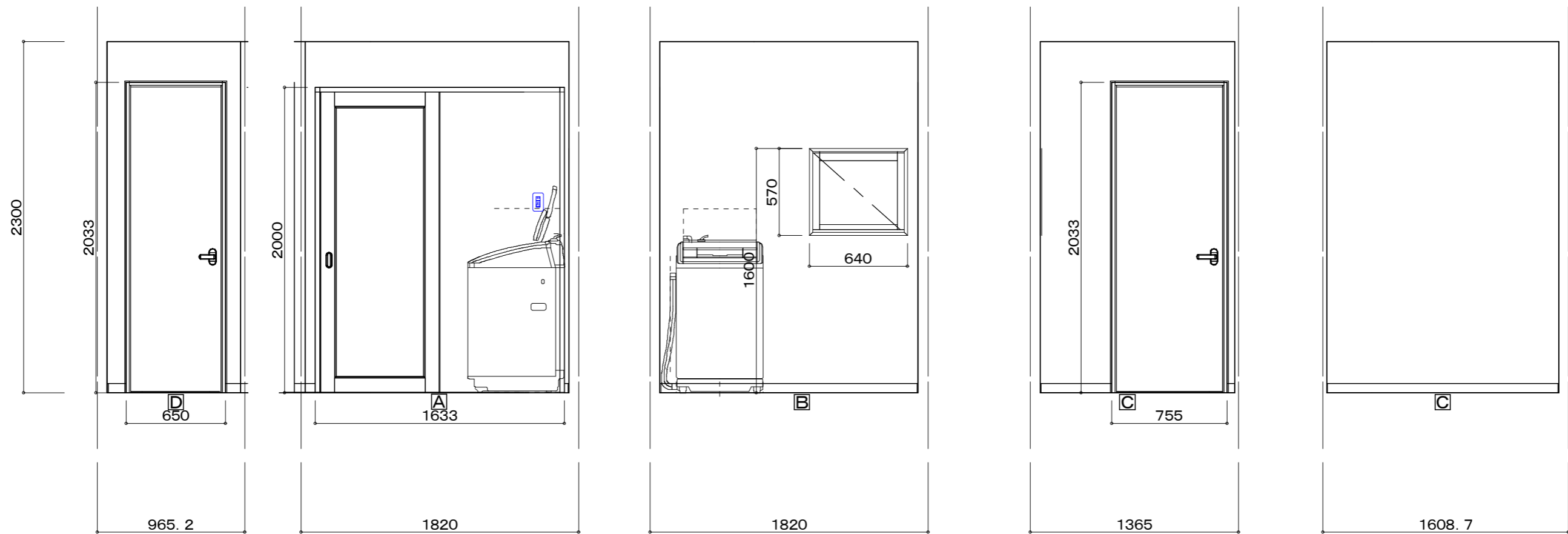
脱衣室展開図
