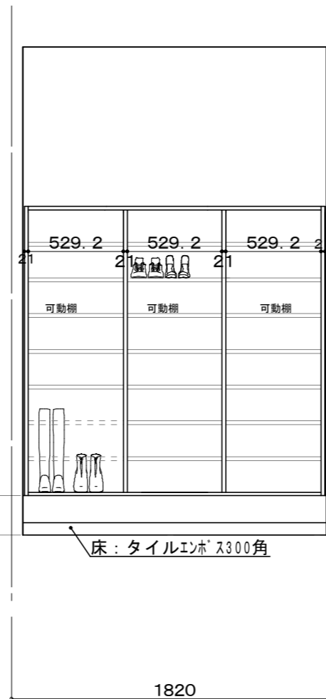
玄関展開図
