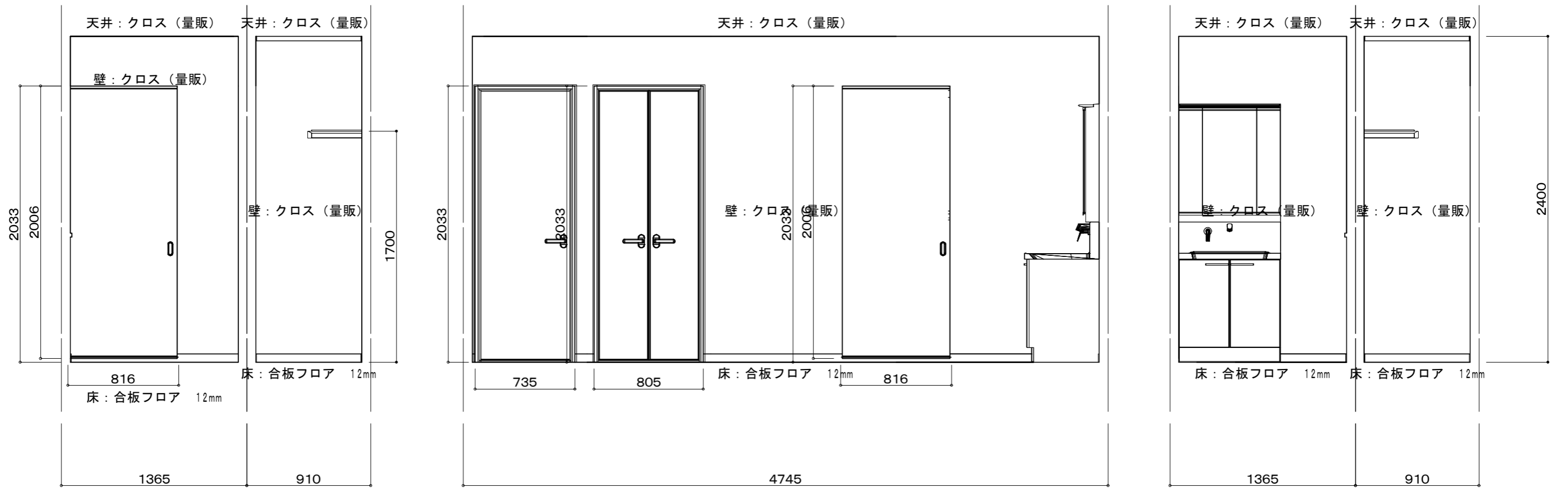
廊下展開図
