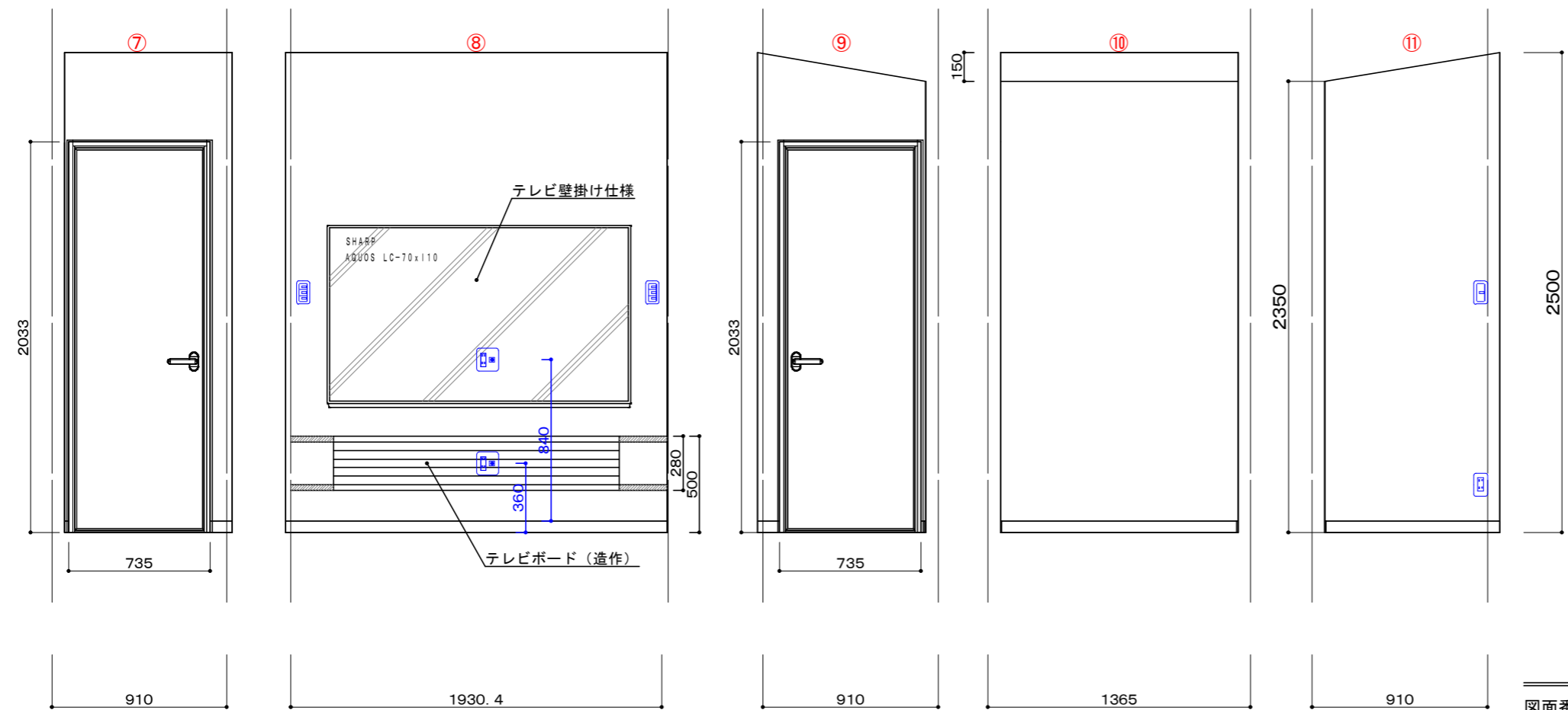
LDK展開図
