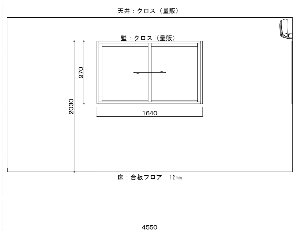
寝室展開図
