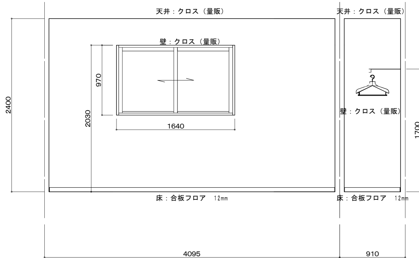
子供室A展開図
