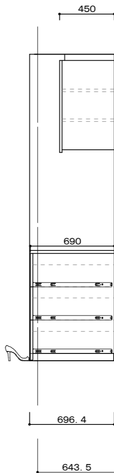
LDK展開図
