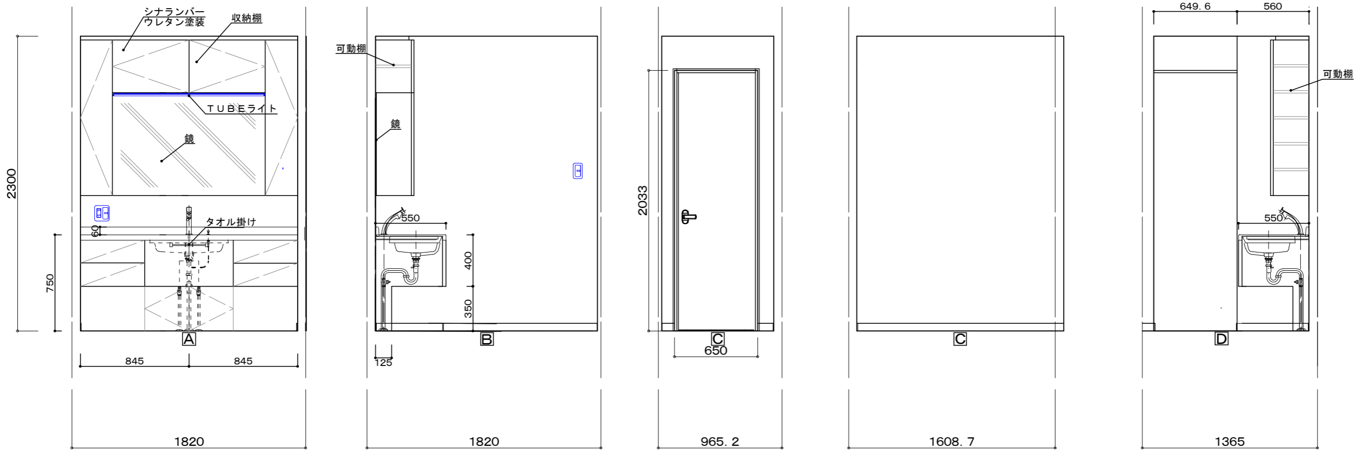
洗面室展開図
