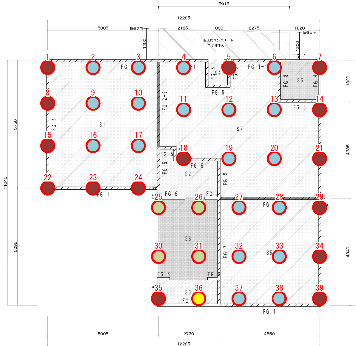
1階：基礎伏図
